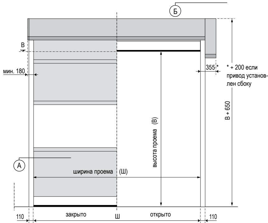
Вид спереди
